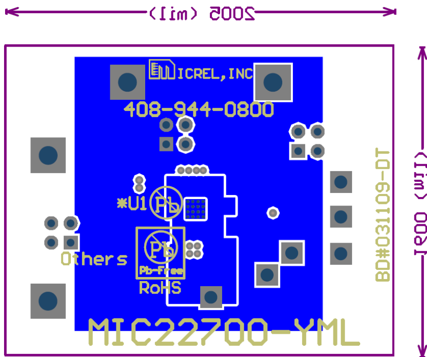
Bottom Layer
