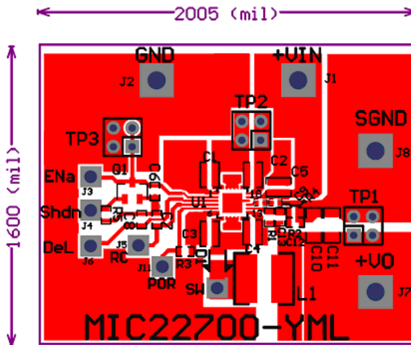
Top Layer
